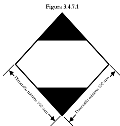
Marca para volumes que contenham quantidades limitadas
