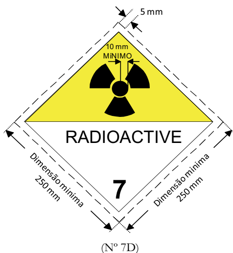
Placa-etiqueta para matérias radioativas da classe 7
