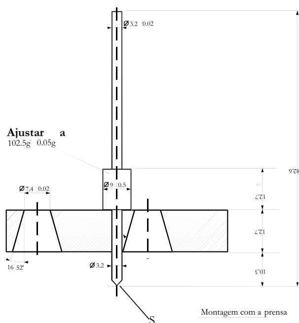
Figura 1 – Penetrómetro
