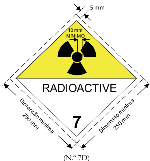
Placa-etiqueta para matérias radioativas da classe 7
