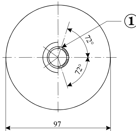
Fig.3: Cilindro oco de bronze, fechado de um lado; Plano e corte vertical, dimensões em mm
