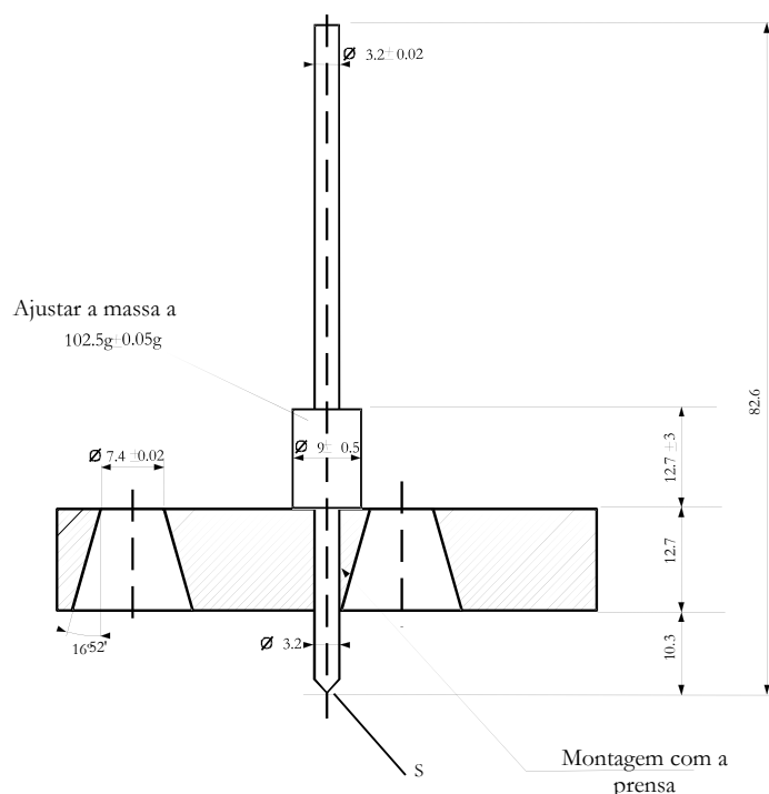
Figura 1 – Penetrómetro
