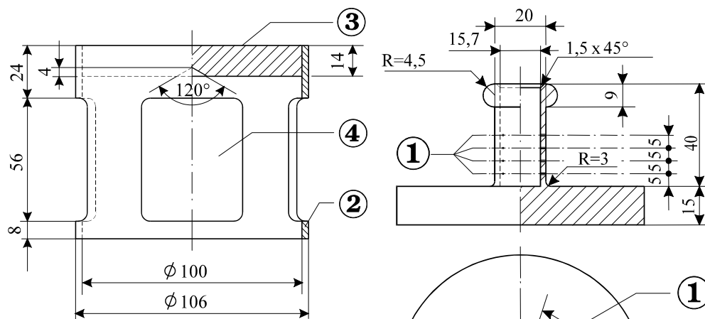
Fig.1: Carga em forma de campânula, massa 2220 g, capaz de ser suspensa sobre o êmbolo de bronze.
