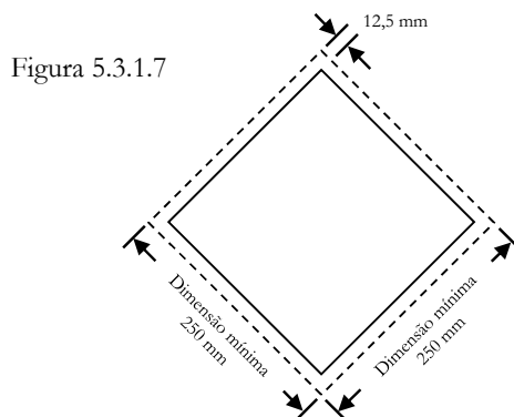
Placa-etiqueta (exceto para a Classe 7)
