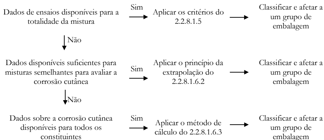
Figura 2.2.8.1.6.1: Abordagem para a classificação e afetação de misturas corrosivas aos grupos de embalagem
