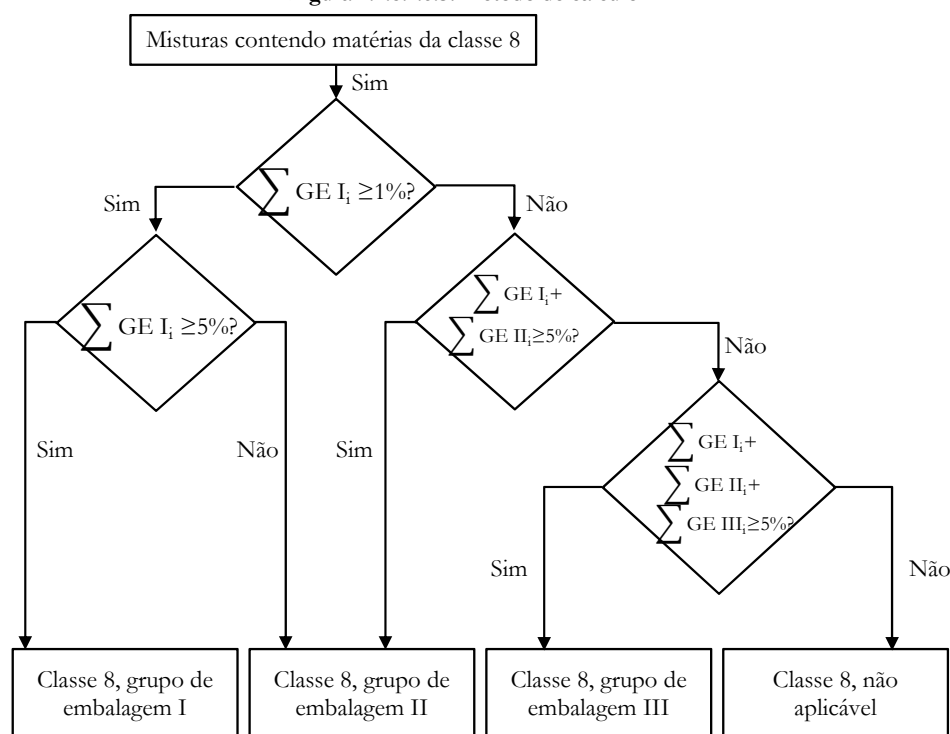
Figura 2.2.8.1.6.3: Método de cálculo
