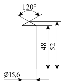
Fig.2: Êmbolo cilíndrico de bronze, dimensões em mm
