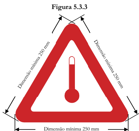
Marca para as matérias transportadas a quente
