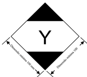
Marca para volumes que contenham quantidades limitadas em conformidade com a Parte 3, Capítulo 4 das Instruções Técnicas da OACI
